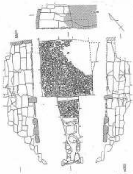
4・下麻生古墳(1号墳)横穴式石室実測図
