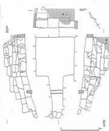
6・下麻生古墳(2号墳)横穴式石室実測図
